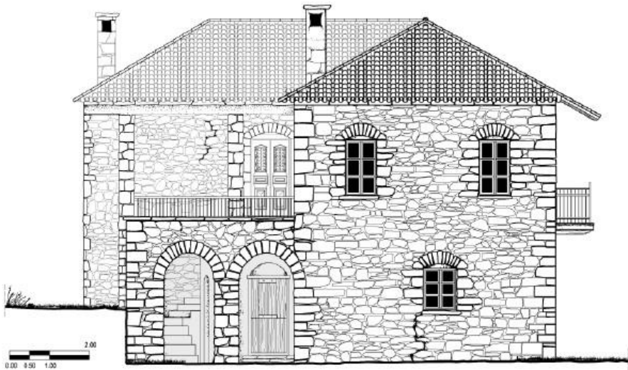
3. Νότια όψη της οικίας Κομπορόζου. Στην αριστερή πλευρά του κτιρίου φαίνεται το λιακωτό και οι θόλοι που το στηρίζουν στο επίπεδο του ισογείου. (Σχέδιο: Μαρία Παπαϊωάννου)
